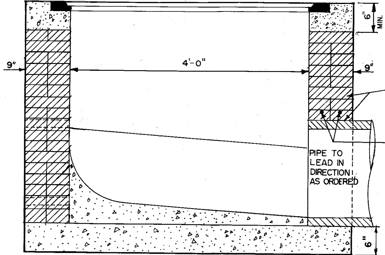
LONGITUDINAL SECTION
